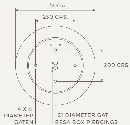
Montageplaat OVIX (afmetingen in mm)
