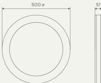
Afschermkap OVIX (afmetingen in mm)
