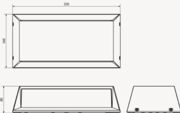
Afschermkap SYMM Plus (afmetingen in mm)
