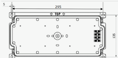
Montageplaat SYMM Plus (afmetingen in mm)
