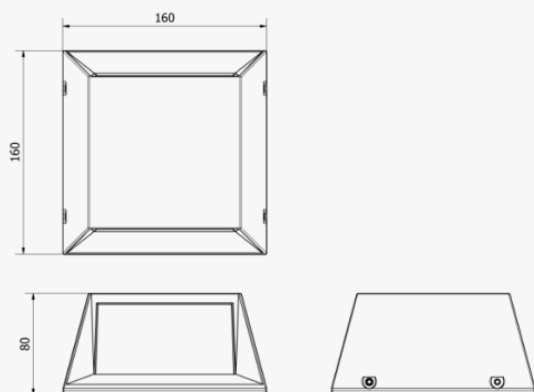
Afschermkap SYMM (afmetingen in mm)
