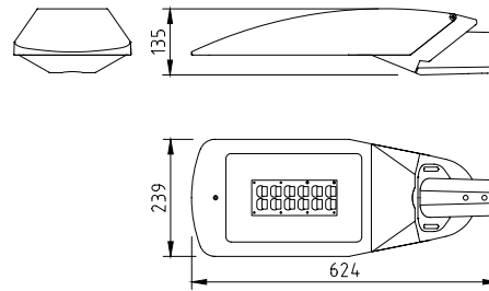
Maststuk 48/60 (opzet)
